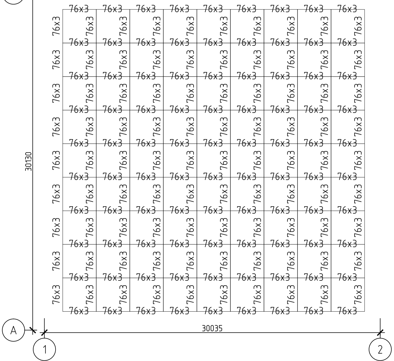
Схема сечений элементов нижнего пояса структурного покрытия №1
