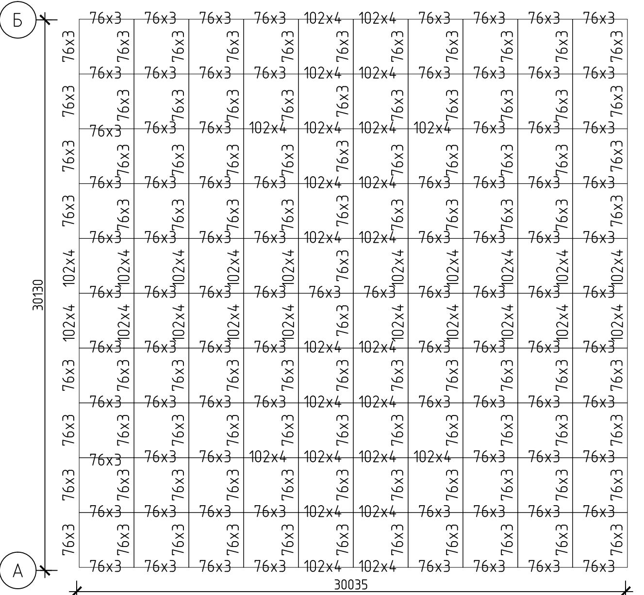
Схема сечений элементов верхнего пояса структурного покрытия №1
